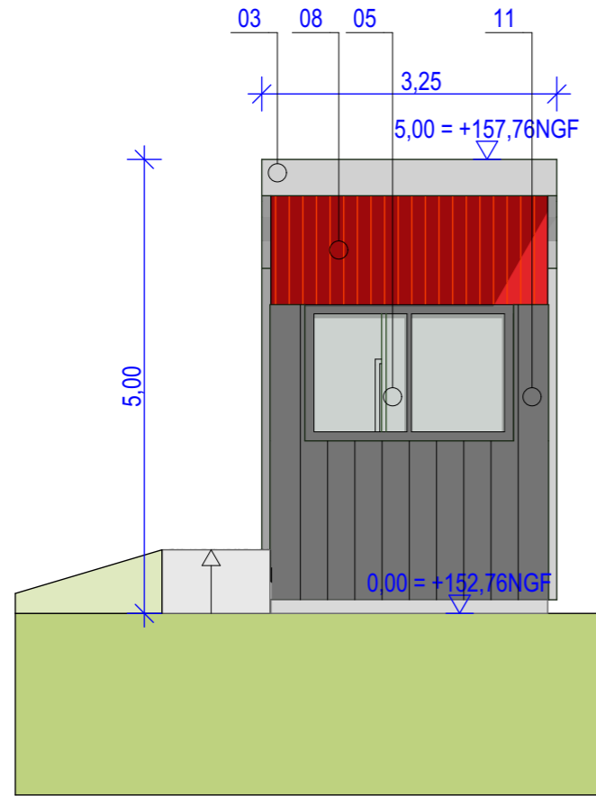
Elevation Nord
