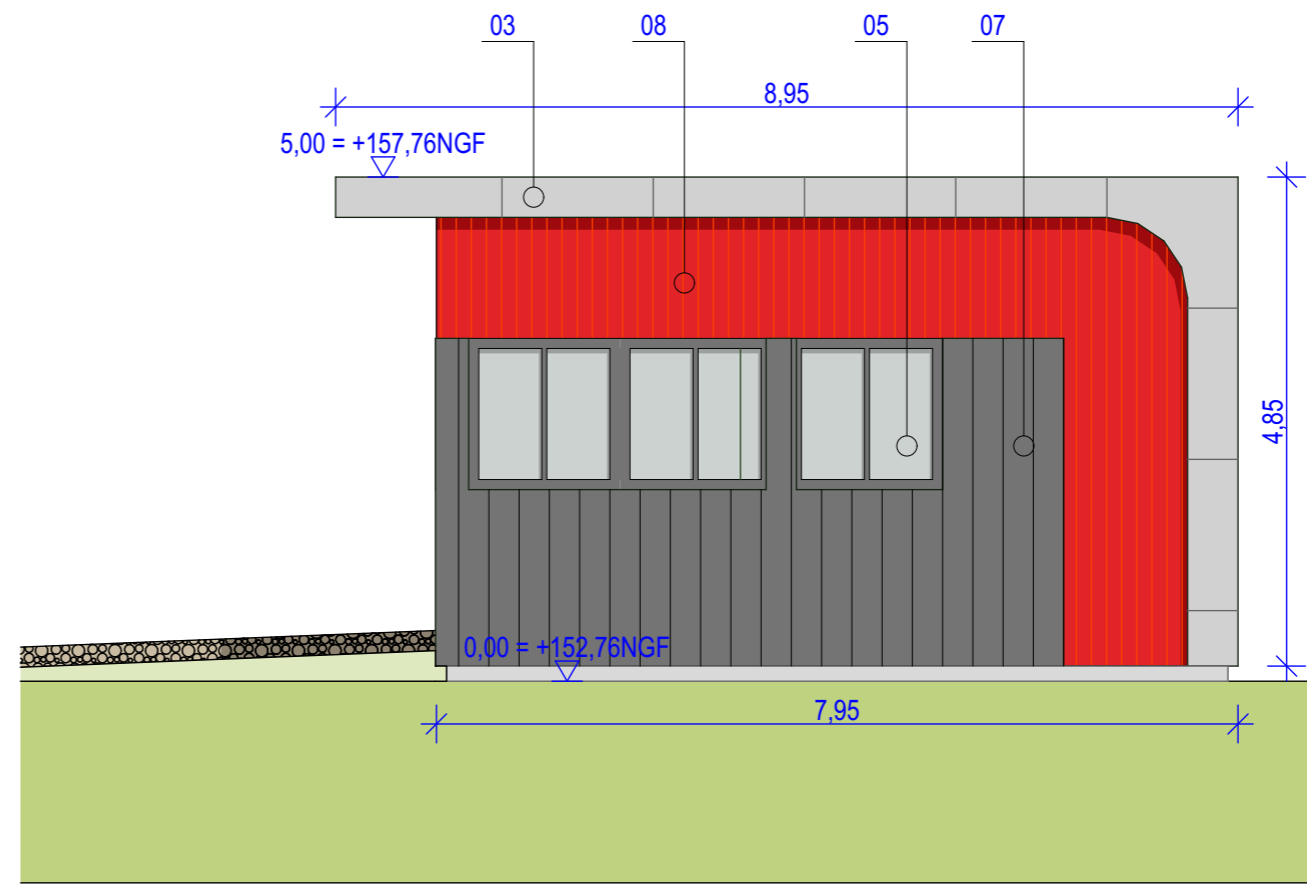
Elevation Ouest
