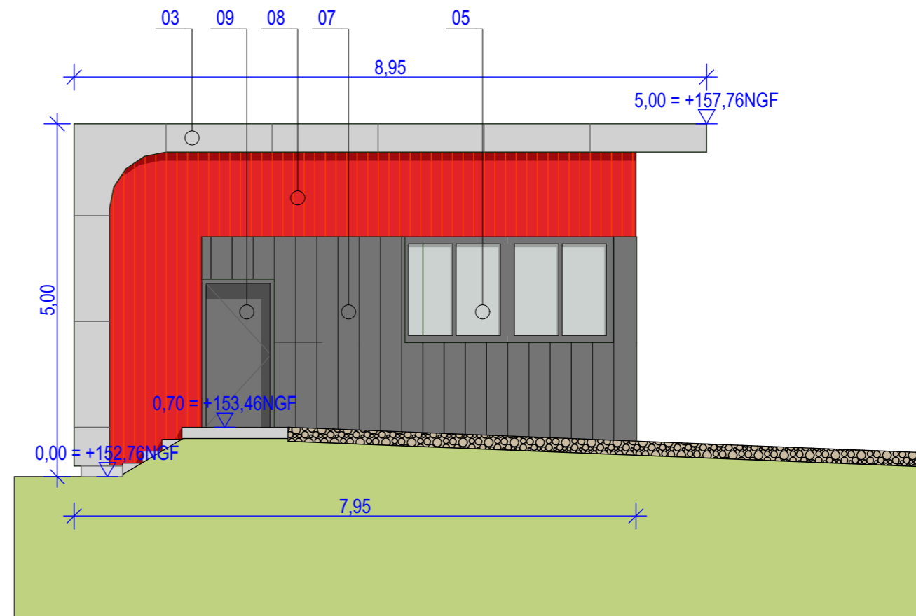
Elevation Est
