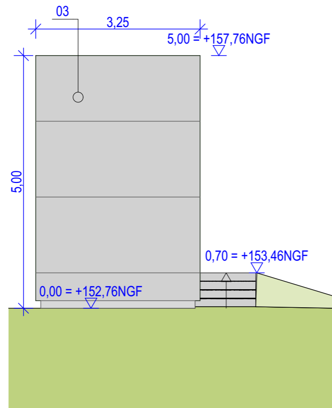
Elevation Sud
