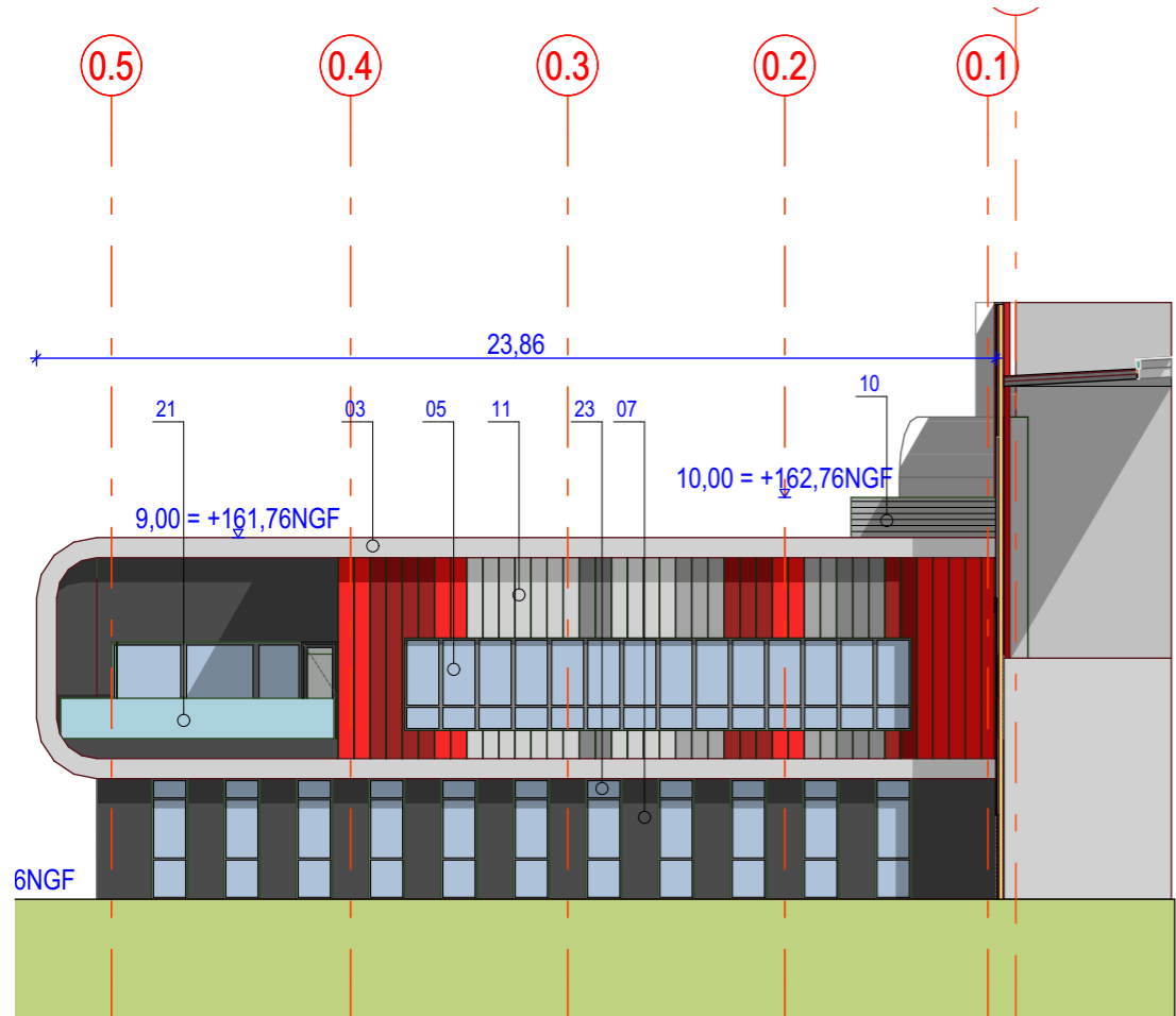
Bureaux 4-5 / Elevation Est
