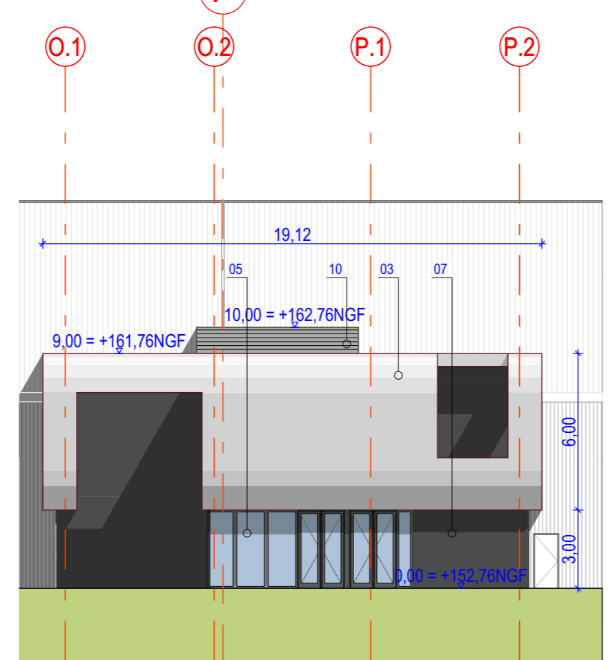
Bureaux 4-5 / Elevation Sud
