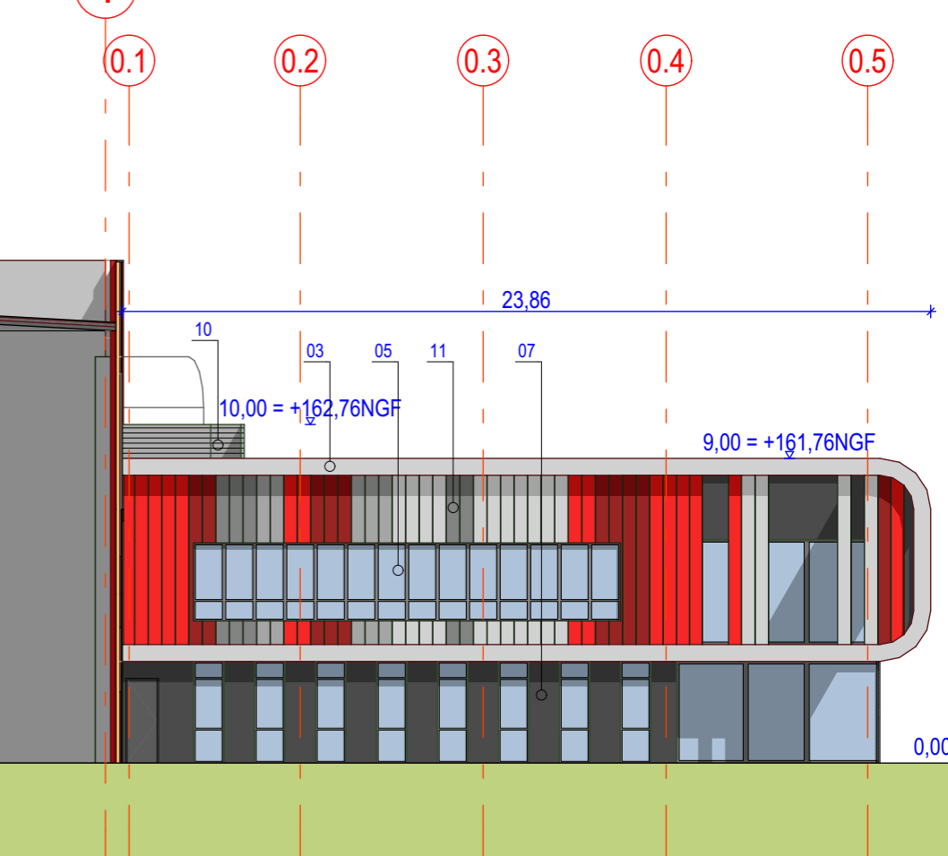
Bureaux 4-5 / Elevation Ouest
