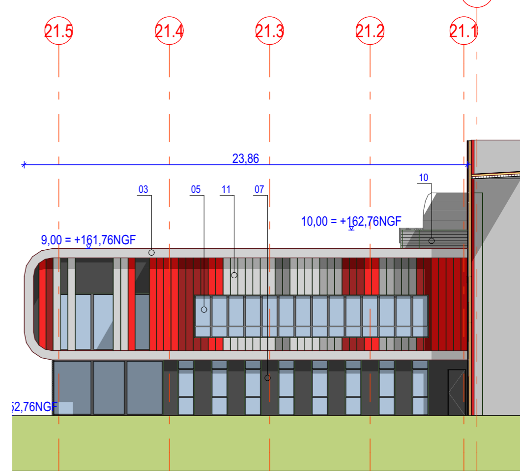
Bureaux 2-3 / Elevation Ouest
