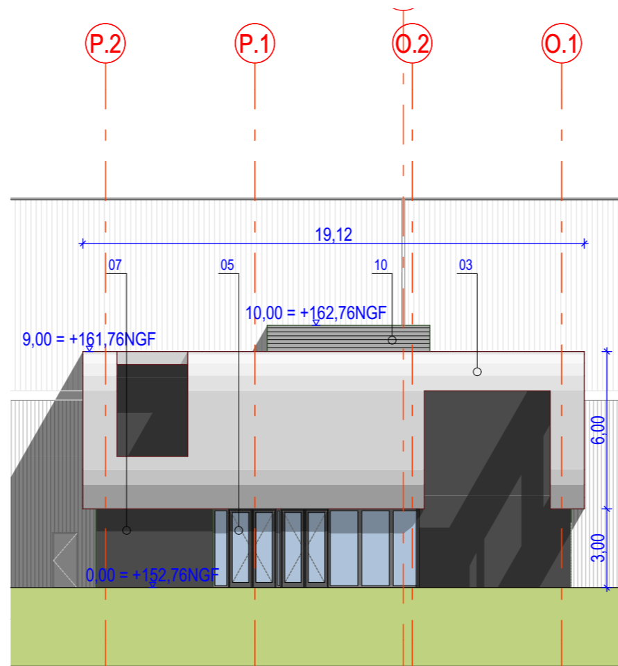
Bureaux 2-3 / Elevation Nord
