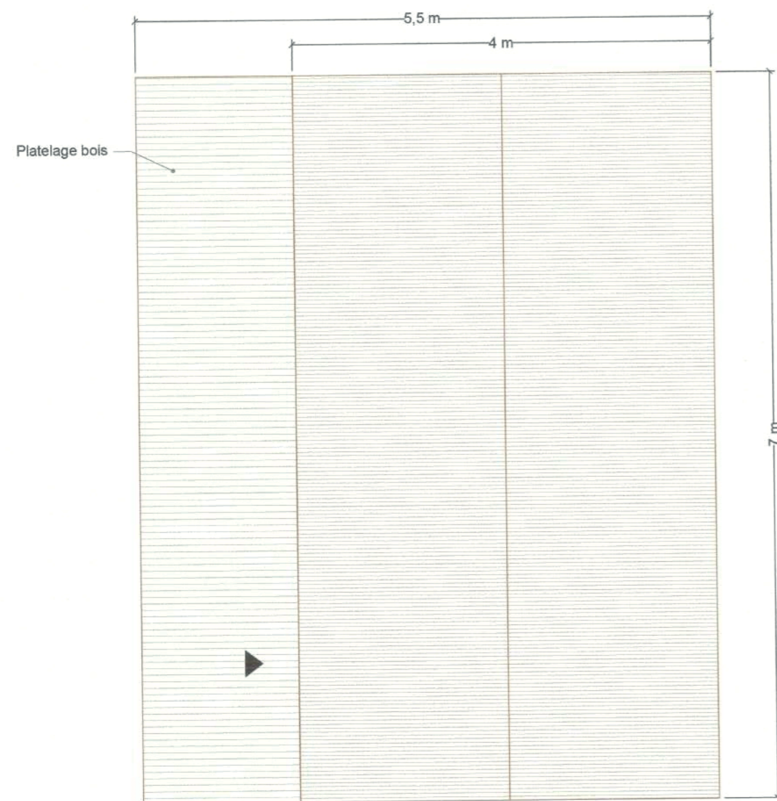
Elévations et plan Echelle 1/50
